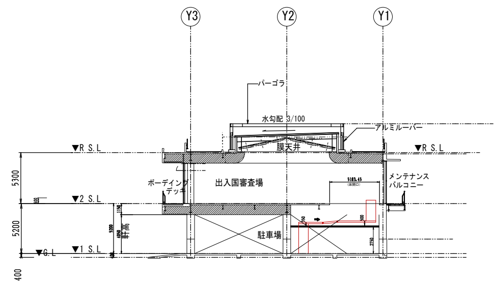
断面図 S-1:200
