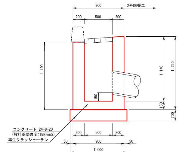
(B)-(B) 断面
