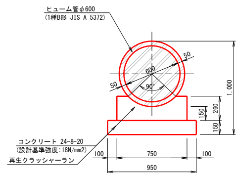
ヒューム管 φ600 90° 固定基礎
