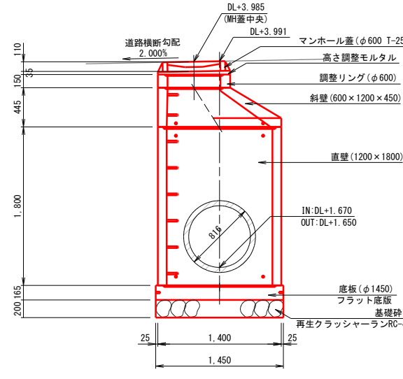
B-B断面図
