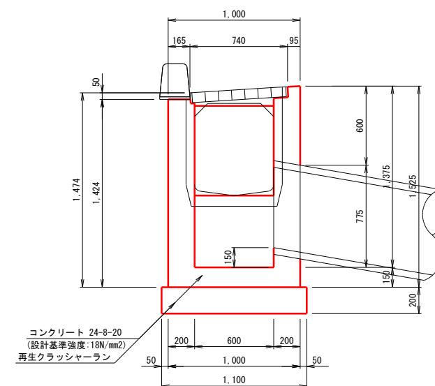
(B)-(B) 断面
