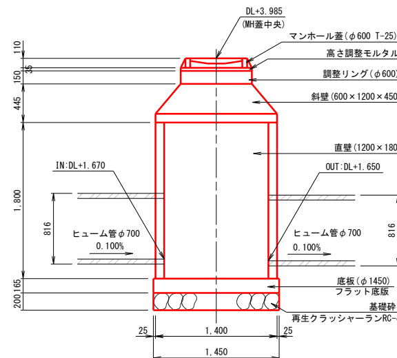
A-A断面図
