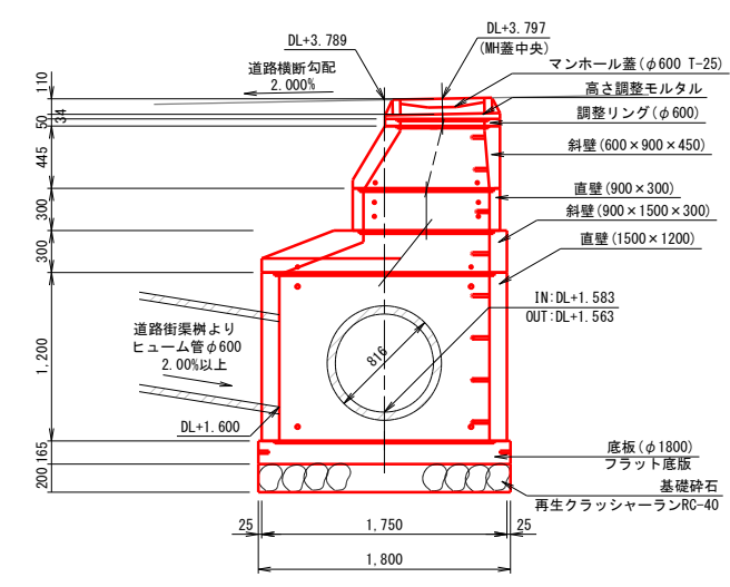
B-B断面図
