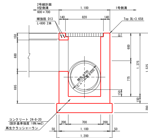
(A)-(A) 断面
