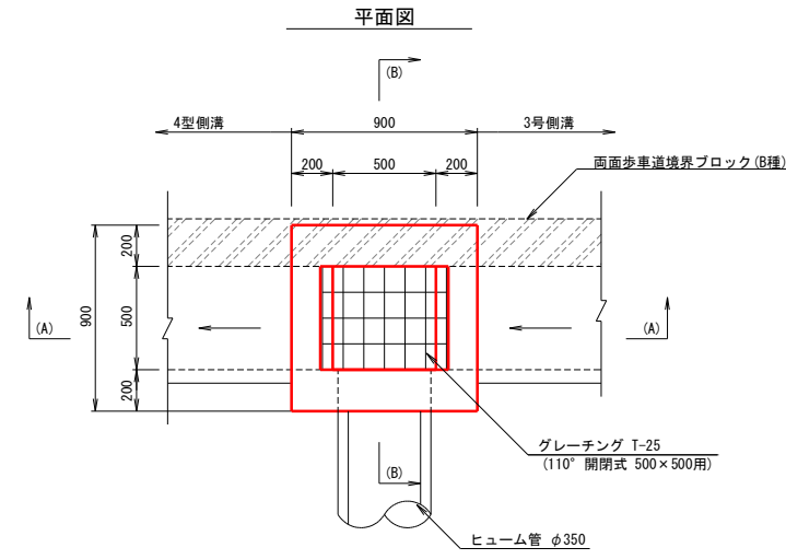
現場打ちグレーチング付き樹
