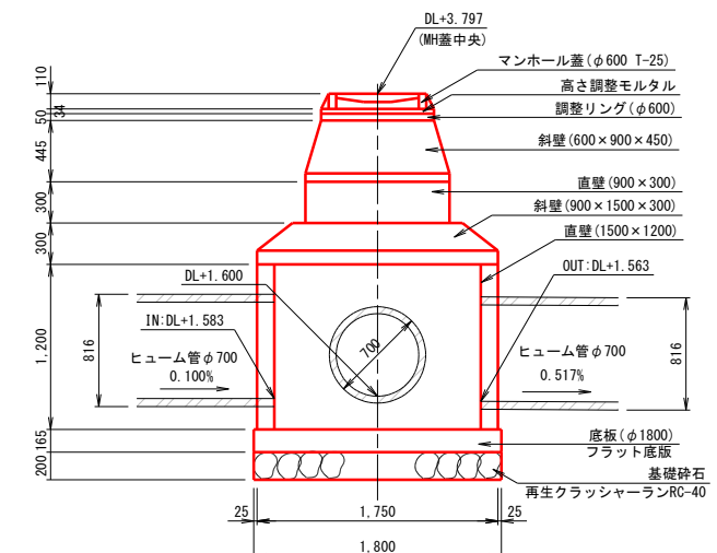
A-A断面図
