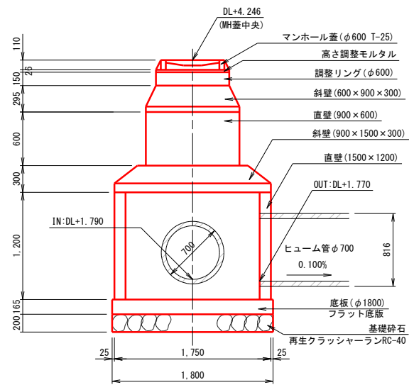
A-A断面図
