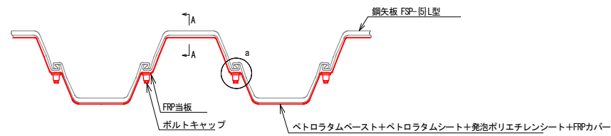
平面図 S=1:15
