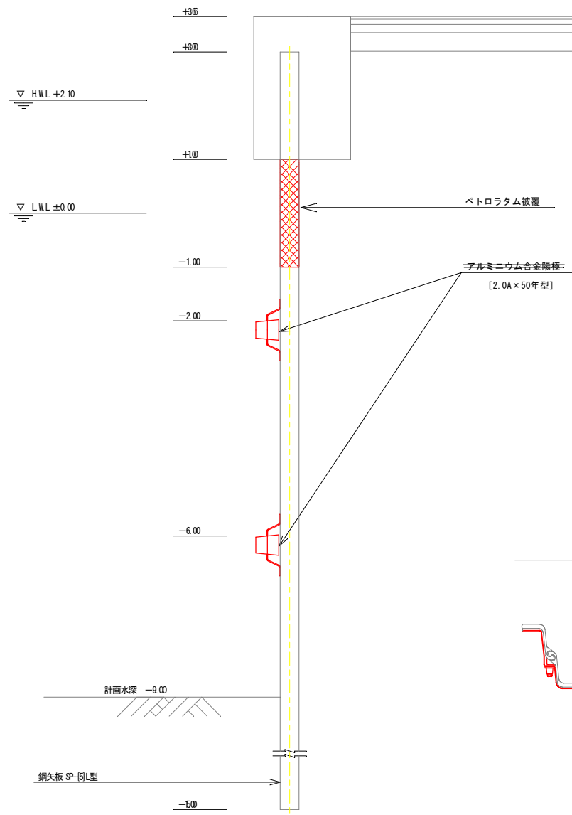
標準断面図 S=1:50
