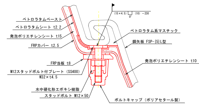
a部詳細図 S=1:2
