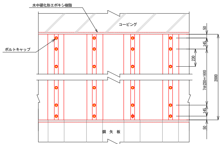
正面図 S=1:15
