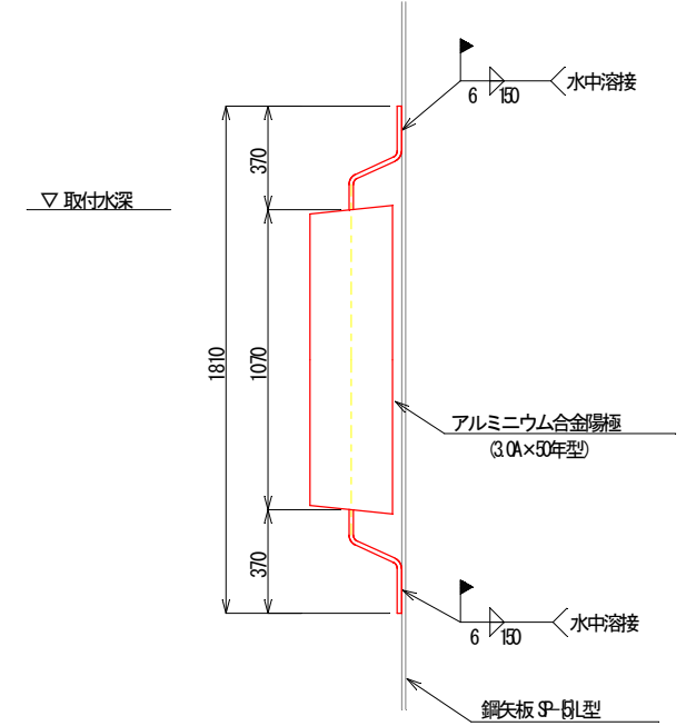
陽極取付詳細図 S=1:15
