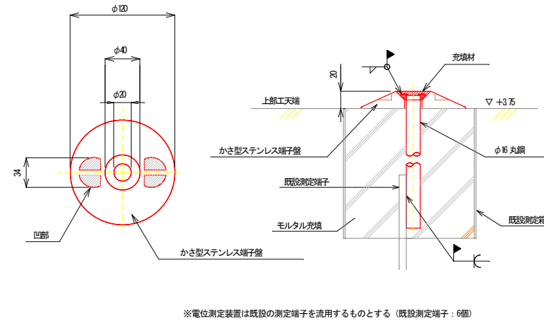
電位測定装置取付要領図 S=1:3
