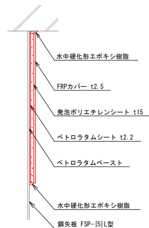
A-A 断面図
