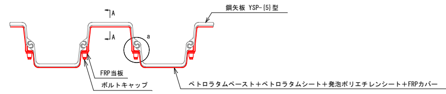
平面図 S=1:15
