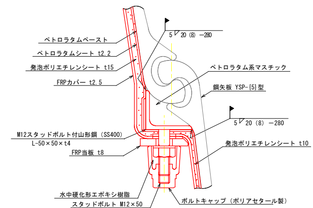
a部詳細図 S=1:2
